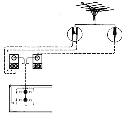
図1 FM専用外部アンテナの接続
