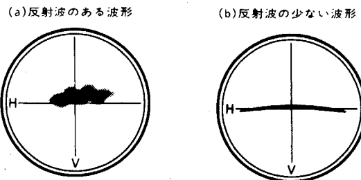
図6 マルチパス波形の観測
